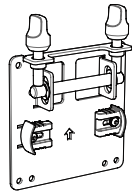
VESA plate (3x)
